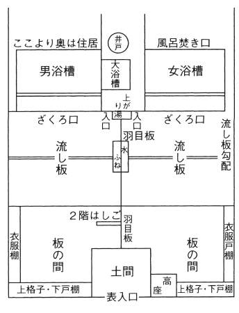
江戸の銭湯の平面図 (『守貞謄稿』より作図)
